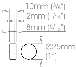
19mm (3/4") stud
