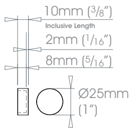
19mm (3/4") Stud
