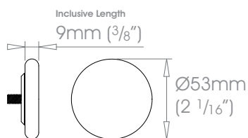
38mm (1 1/2") Classic - Stud
