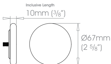
50mm (2") Classic - Stud
