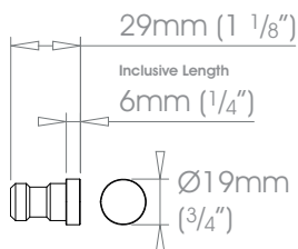
19mm (3/4") Flush Stud
